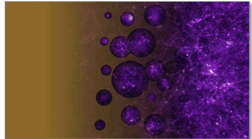
cosmic reionisation
